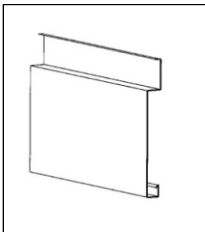
Panel poziomy HZ, niedeklowany, fuga stała 20 mm, szerokość osiowa panela = widoczna część panela + 2 × ½ fugi, dł. stand. 3 lub 4 m
