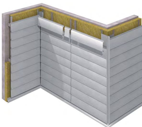
Panel nakładkowy ST
